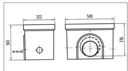
Gyűjtőakna rövid alsó rész
