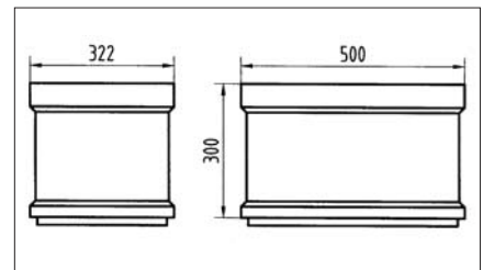
Gyűjtőakna közbenső rész
