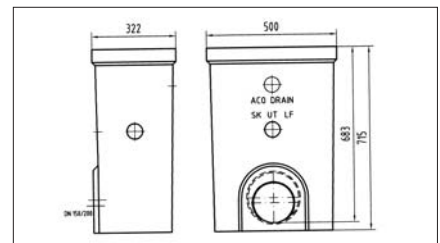
Gyűjtőakna hosszú alsó rész
